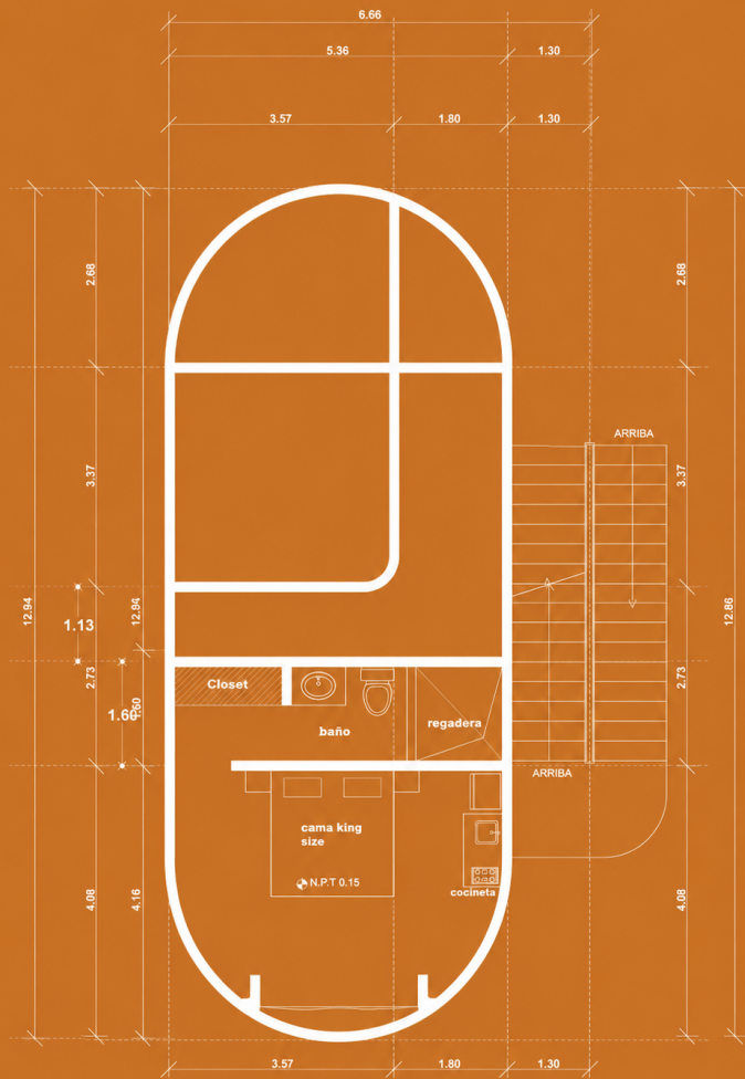
PLANTA ARQUITECTÓNICA BAJA
