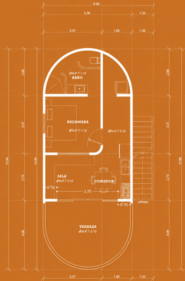
PLANTA ARQUITECTÓNICA PRIMER NIVEL
