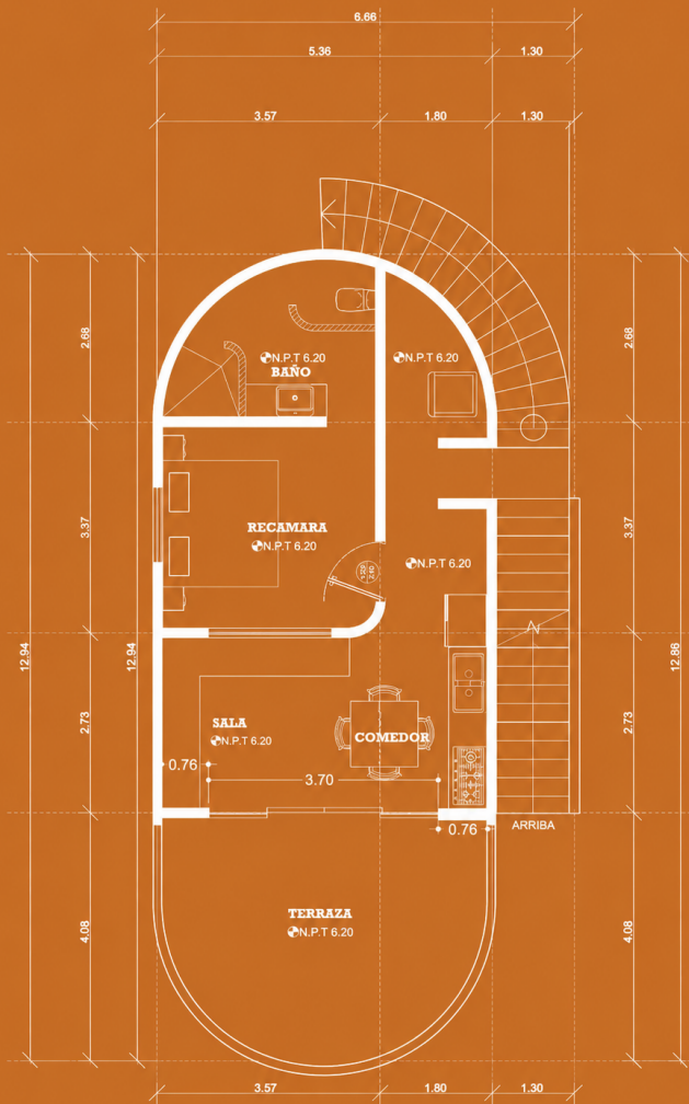
PLANTA ARQUITECTÓNICA SEGUNDO NIVEL
